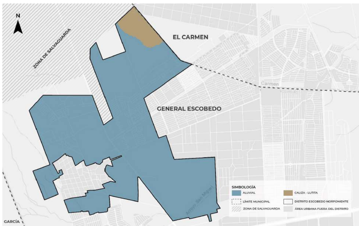
Figura 12. Geología.
