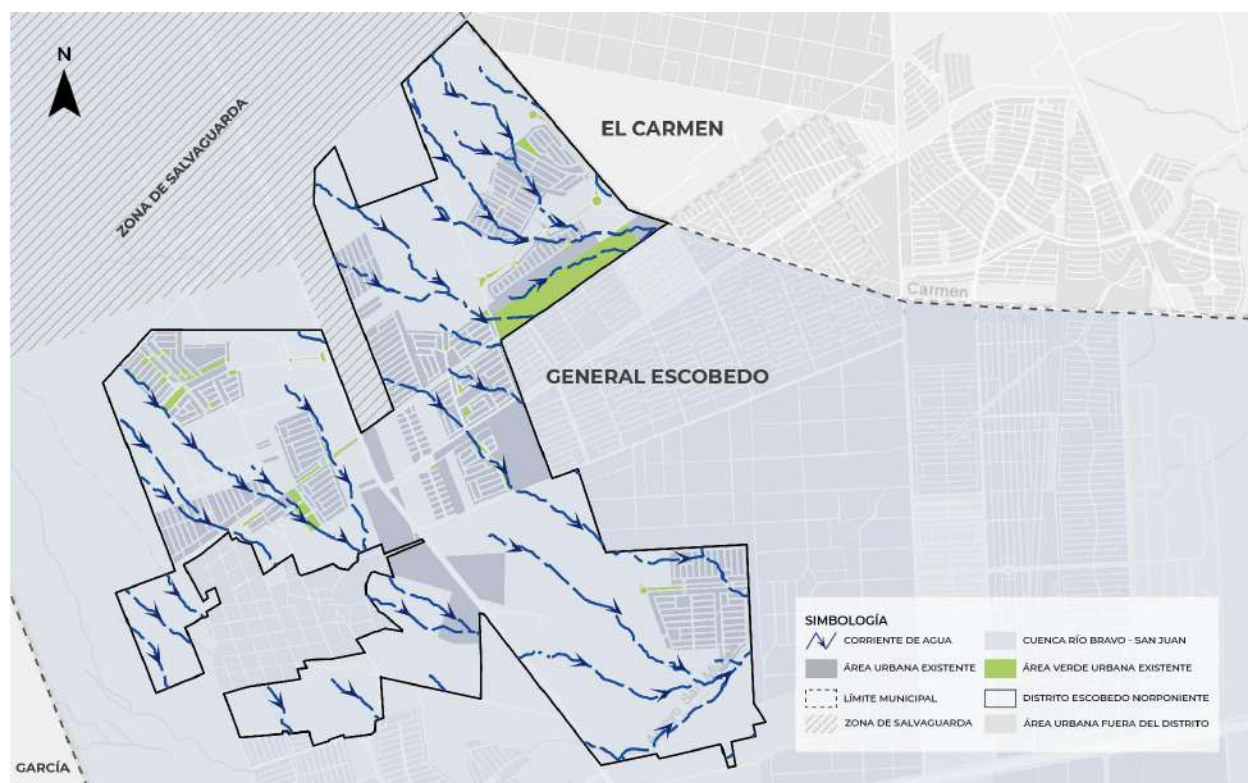
Figura 15. Hidrología.
